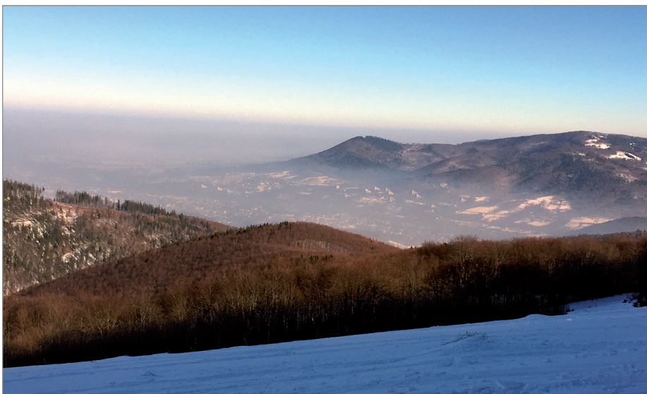
Smog nad Ustroniem widoczny z Poniwca.
