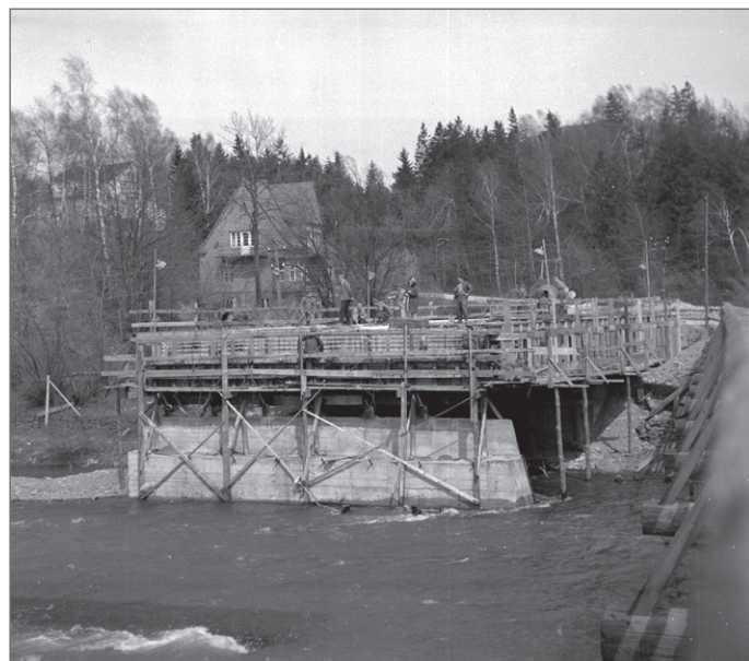
Budowa mostu na Zawodzie.
