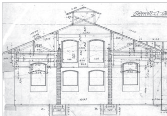
Przekrój budynku Huty „Klemensa” widocznej od północy.
