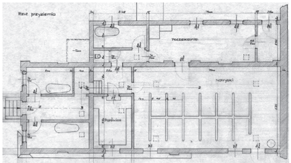
Plan kąpielarni, sporządzony 10 marca 1947 r.
