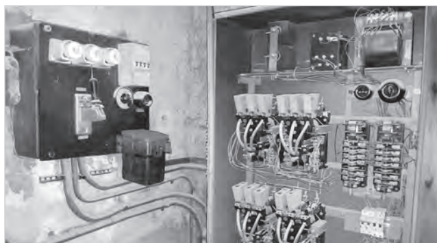
Zmodernizowana skrzynka rozdzielcza windy.
