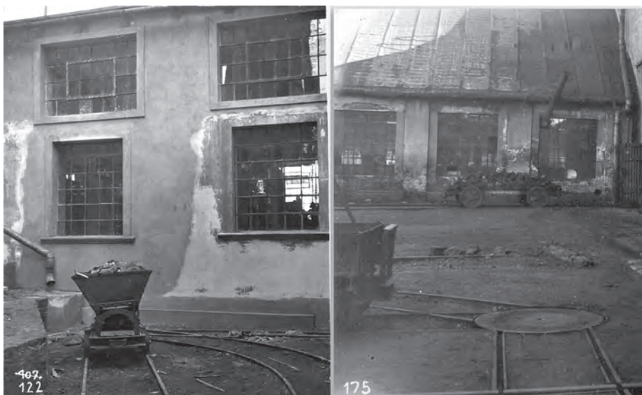
Elementy kolei wąskotorowej w Kuźni na unikalnych ujęciach z lat 30. XX w.. Z lewej koliba z fragmentami torów, z prawej obrotnica.
