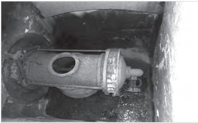
Wnętrze komory wraz z niemal kompletną turbiną w podziemiu obecnego Zespołu Szkół Technicznych.
