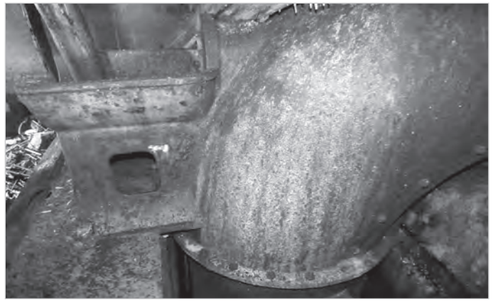
Relikty pod ustronską Kuźnią: krzywak - kolano łączące turbinę z rurą ssawką, przez które przechodził poziomo jej wał oraz element ułożyskowania wału.
