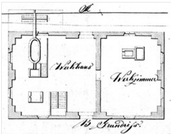
Pierwotny rozkład pomieszczeń papierni w Hermanicach na planie z 1837 r. Z lewej zakład z kołem wodnym, z prawej pracownia rzemieślnicza.
