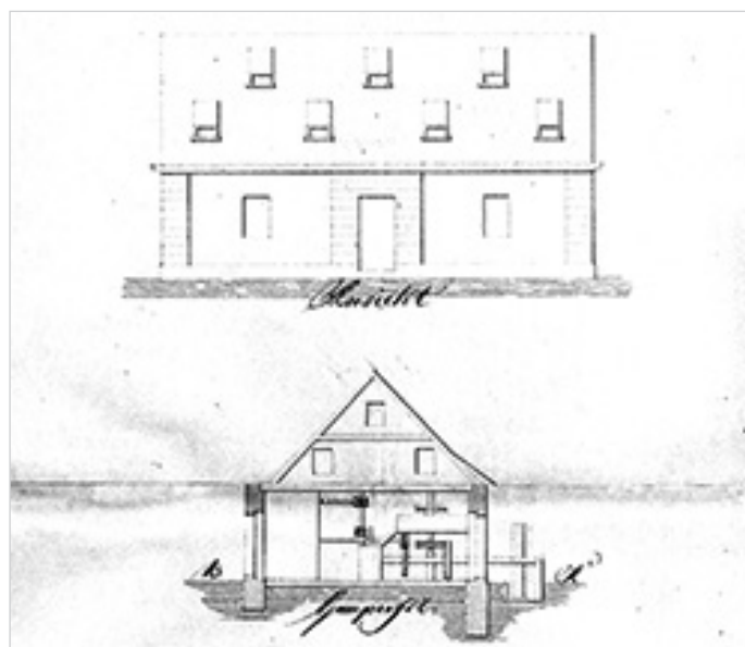
U góry front budynku papierni w Hermanicach, z dołu jego przekrój poprzeczny z widocznym układem kół zębatach, przenoszących napęd z wału koła wodnego na maszyny. Z prawej przekrój kanału Młynówka z widocznym kołem wodnym podsiębiernym.
